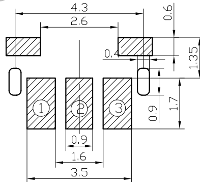
安装参考图
