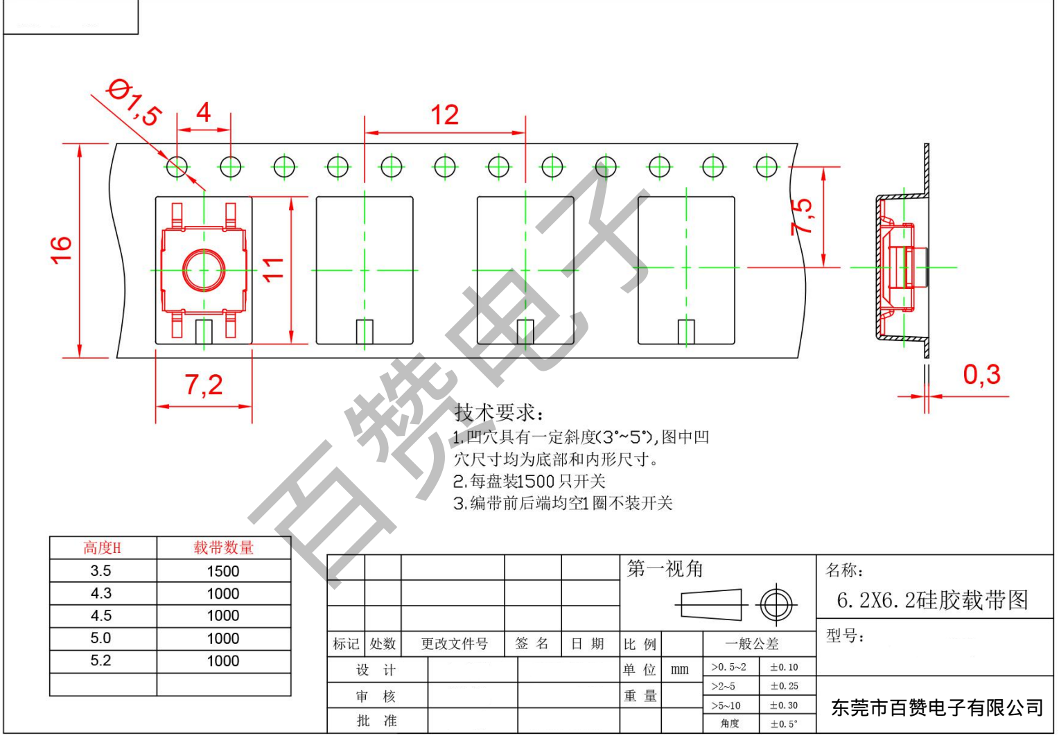
10. Taping diagram 编带示意图:
