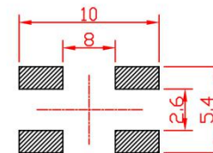
PCB. 焊接图
