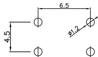
安装参考图
